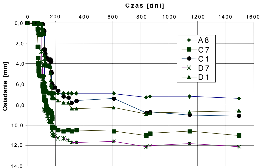
Rys. 4 Obserwowane osiadanie reperów kontrolnych pokazanych na rys. 2a w czasie robót iniekcyjnych oraz po ich zakończeniu (pomiar wykonany przez prof. A. Zurowskiego z zespołem w latach 1995-2000, Politechnika Gdańska, Wydział BWiŚ).
