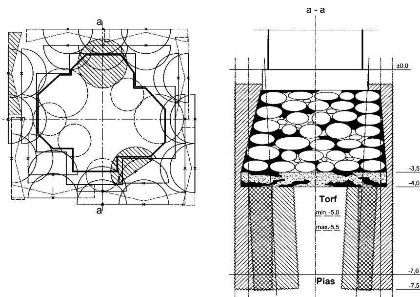
Rys. 3 Rozmieszczenie kolumn, półkolumn i lameli iniekcyjnych pod fundamentem filara C7.
